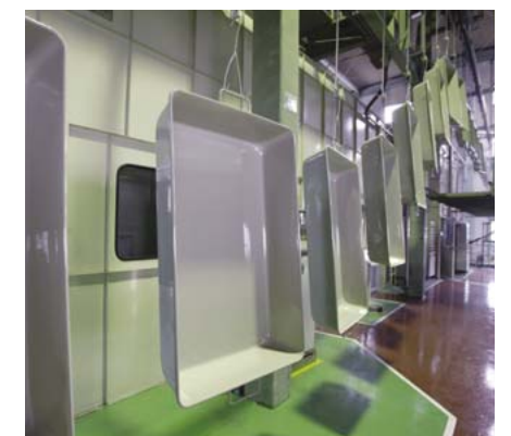
塗装自動順送コンベア
